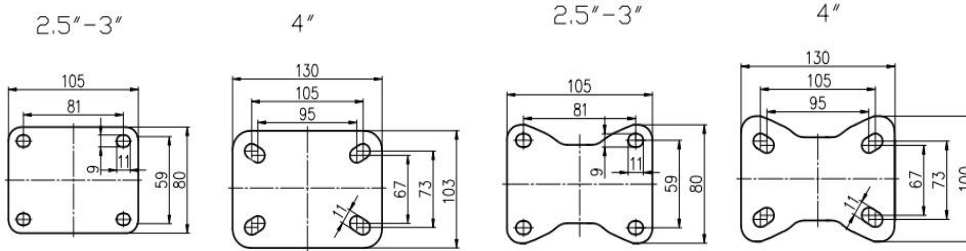
平板万向/刹车
